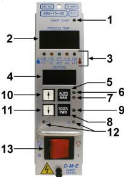
Figure 2 - DSS-15-02 Module
